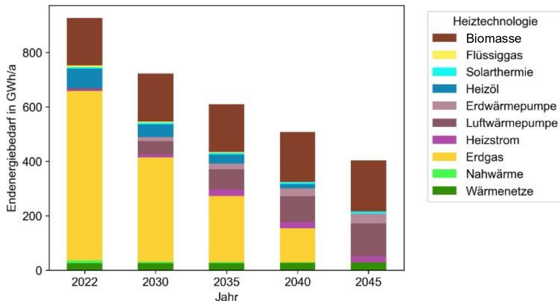
Abbildung 66: Transformation der Endenergiebedarfsdeckung bis 2045
